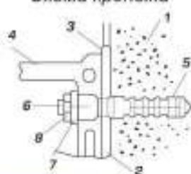
Схема крепежа
